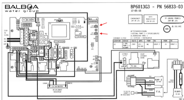
Diagram over Balboa-styring (BP6013G3). De røde pile viser stikkene J34 og J35, hvor CMS-modulets ledning skal placeres.
